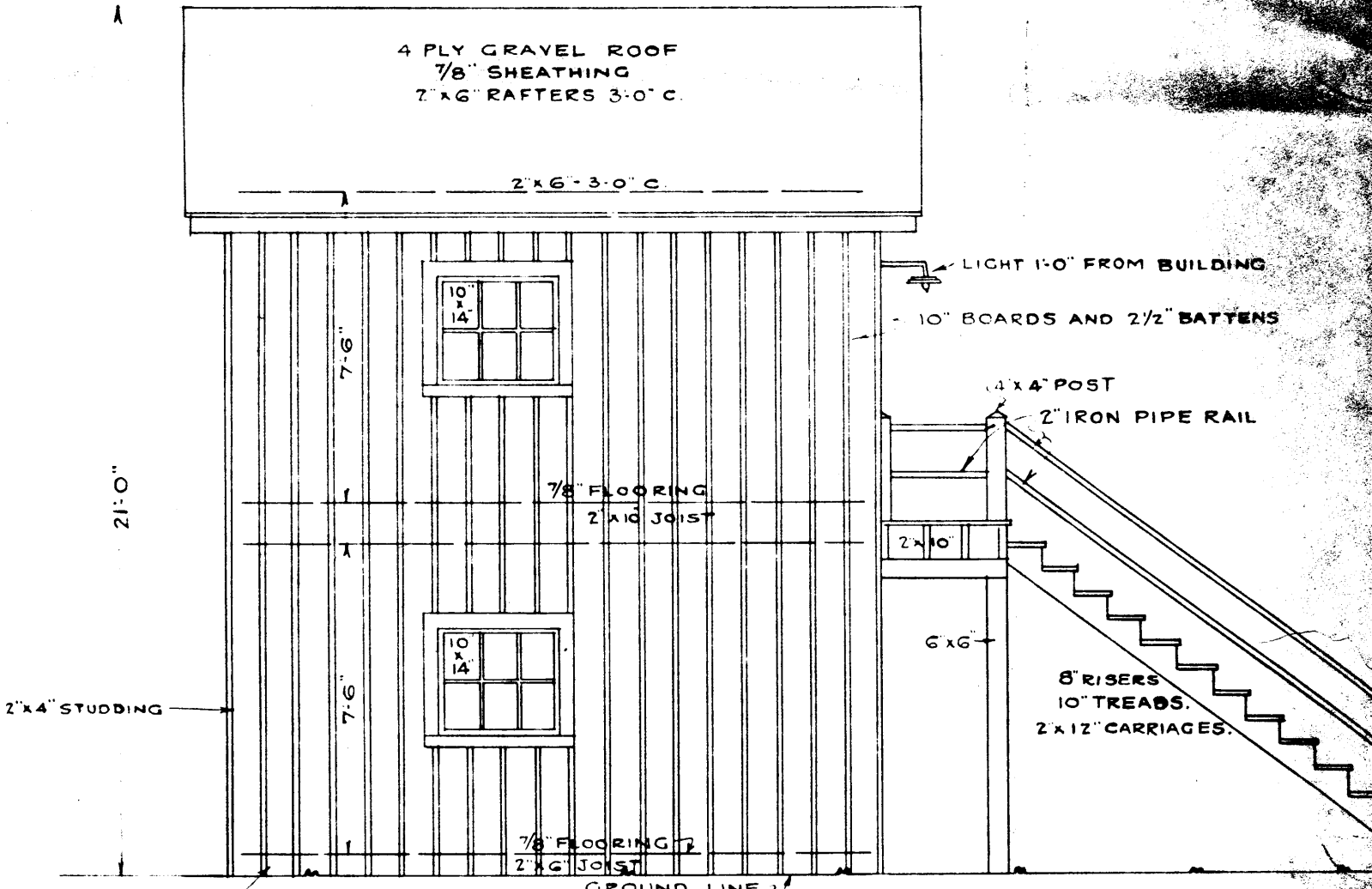
SIDE ELEVATION Scale: 1/4" = 1'-0"
